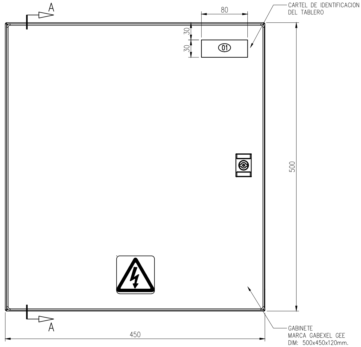
VISTA FRONTAL CON PUERTA (ESC.: 1:4)
