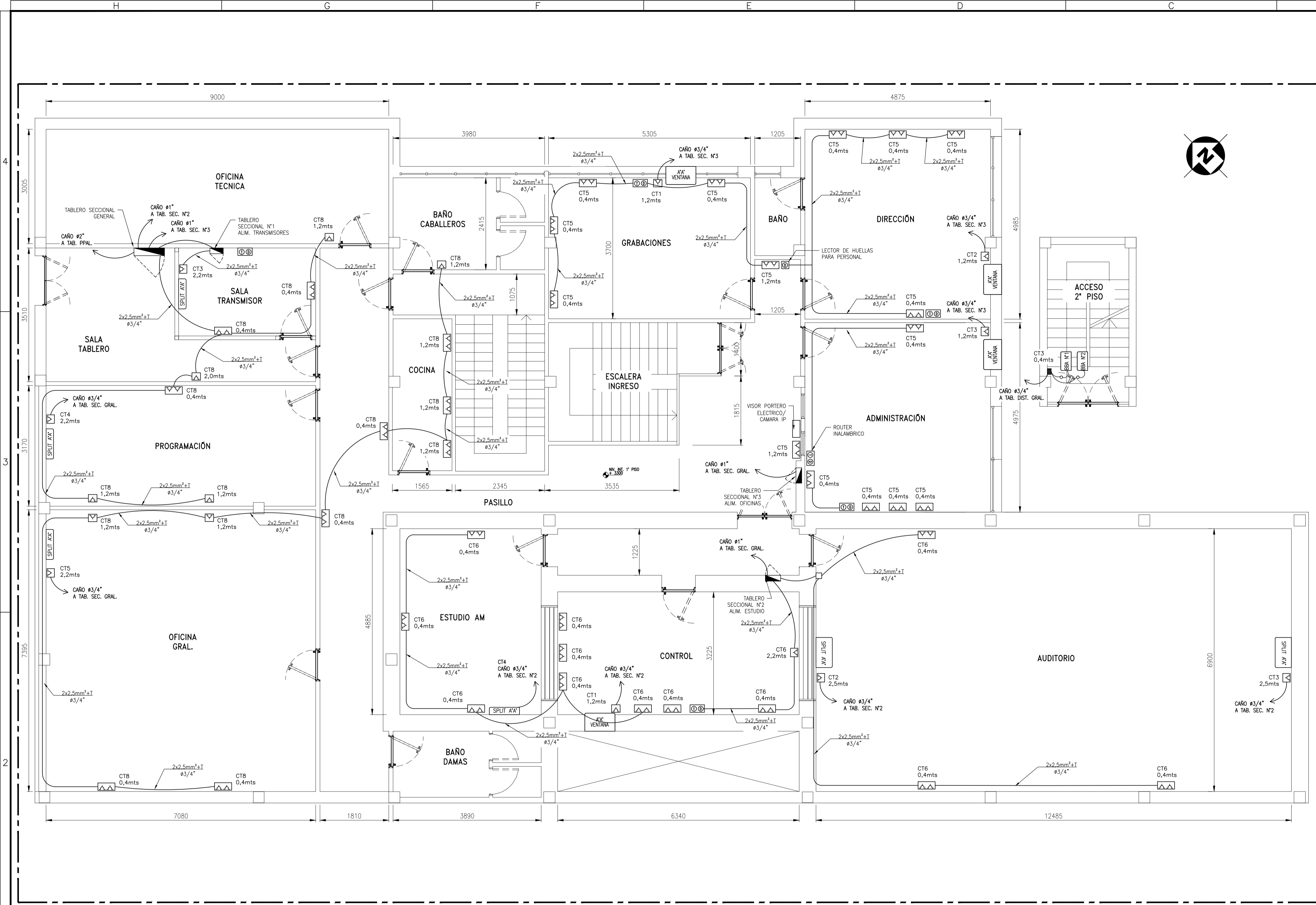
PLANTA 1° PISO SC.1:50
