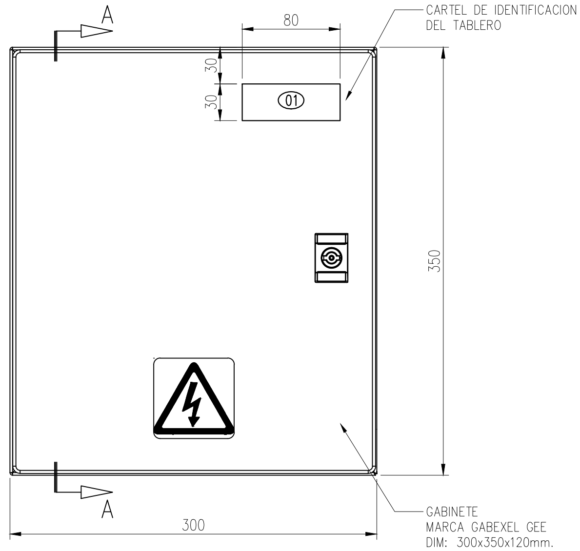
VISTA FRONTAL CON PUERTA (ESC.: 1:4)
